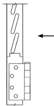
Louver UP
